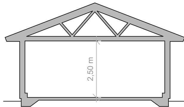
SEKTION
